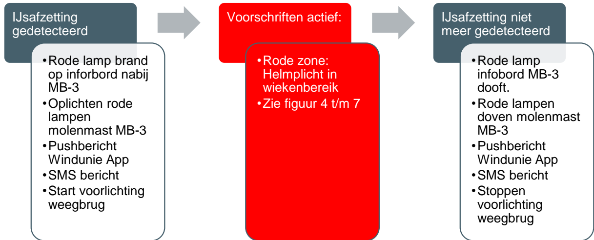
Figuur 3: Stroomschema Icing safety protocol
